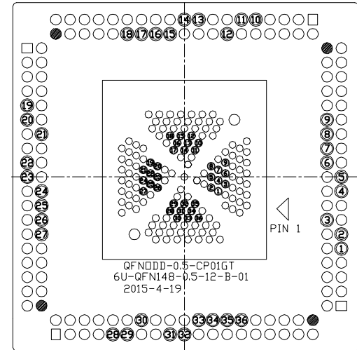
IC 脚位图
